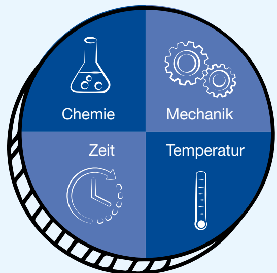
Sinnerscher Kreis
